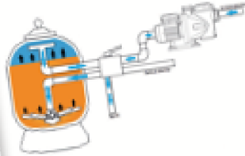
LAVAGE l'eau passe dans le filtre de bas en haut et s'évacue vers l'égout
