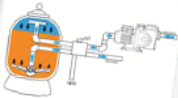
FILTRATION l'eau passe dans le filtre de haut en bas et retourne à la piscine
