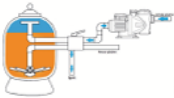
EGOUT l'eau ne passe pas dans le filtre et s'évacue vers l'égout perme de vider la piscine
