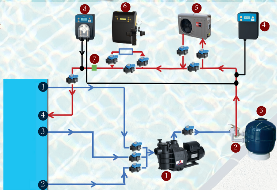
CIRCULATION l'eau ne passe pas dans le filtre et retourne à la piscine permet de brasser la piscine
