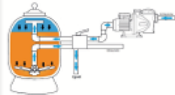
RINCAGE l'eau passe dans le filtre de haut en bas et s'évacue vers l'égout
